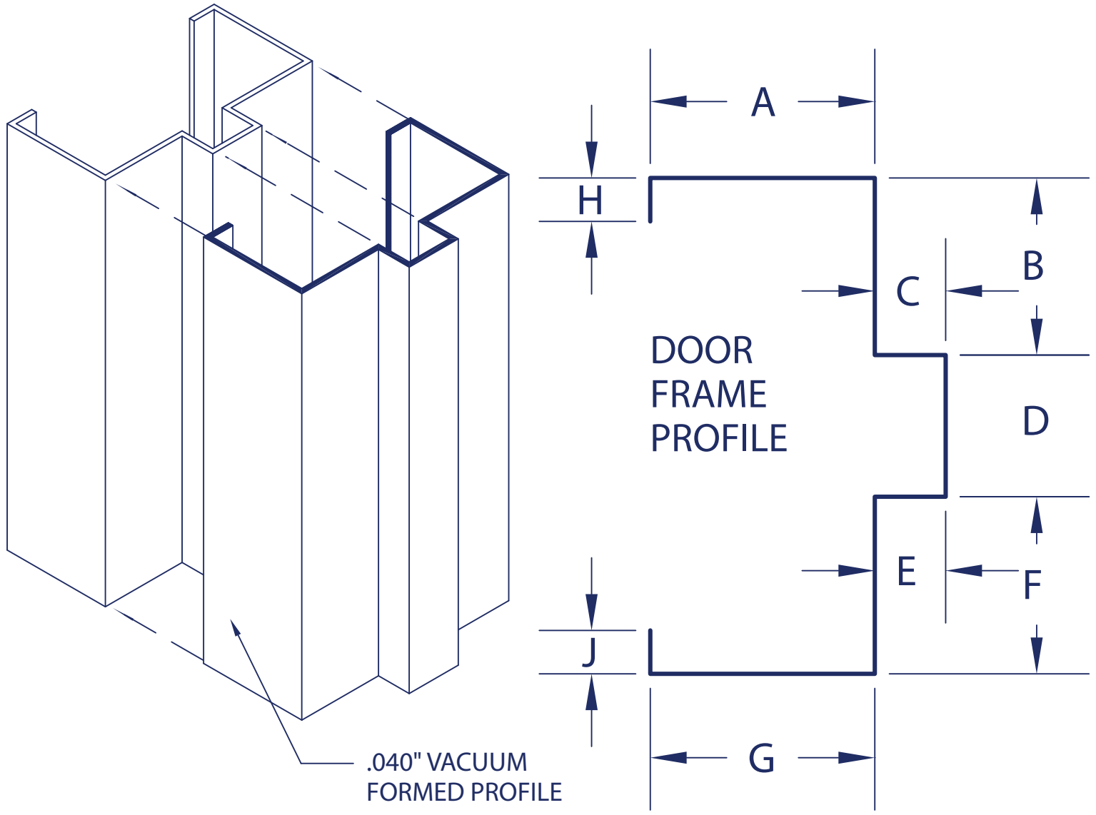
F104, DOOR PROTECTION SCALE: NTS
